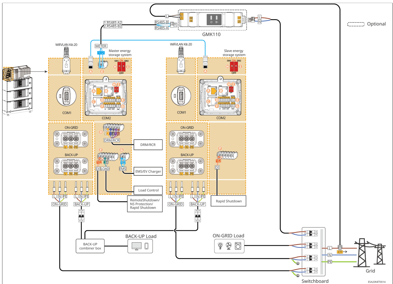
Figuur29 Scenario met GMK110
