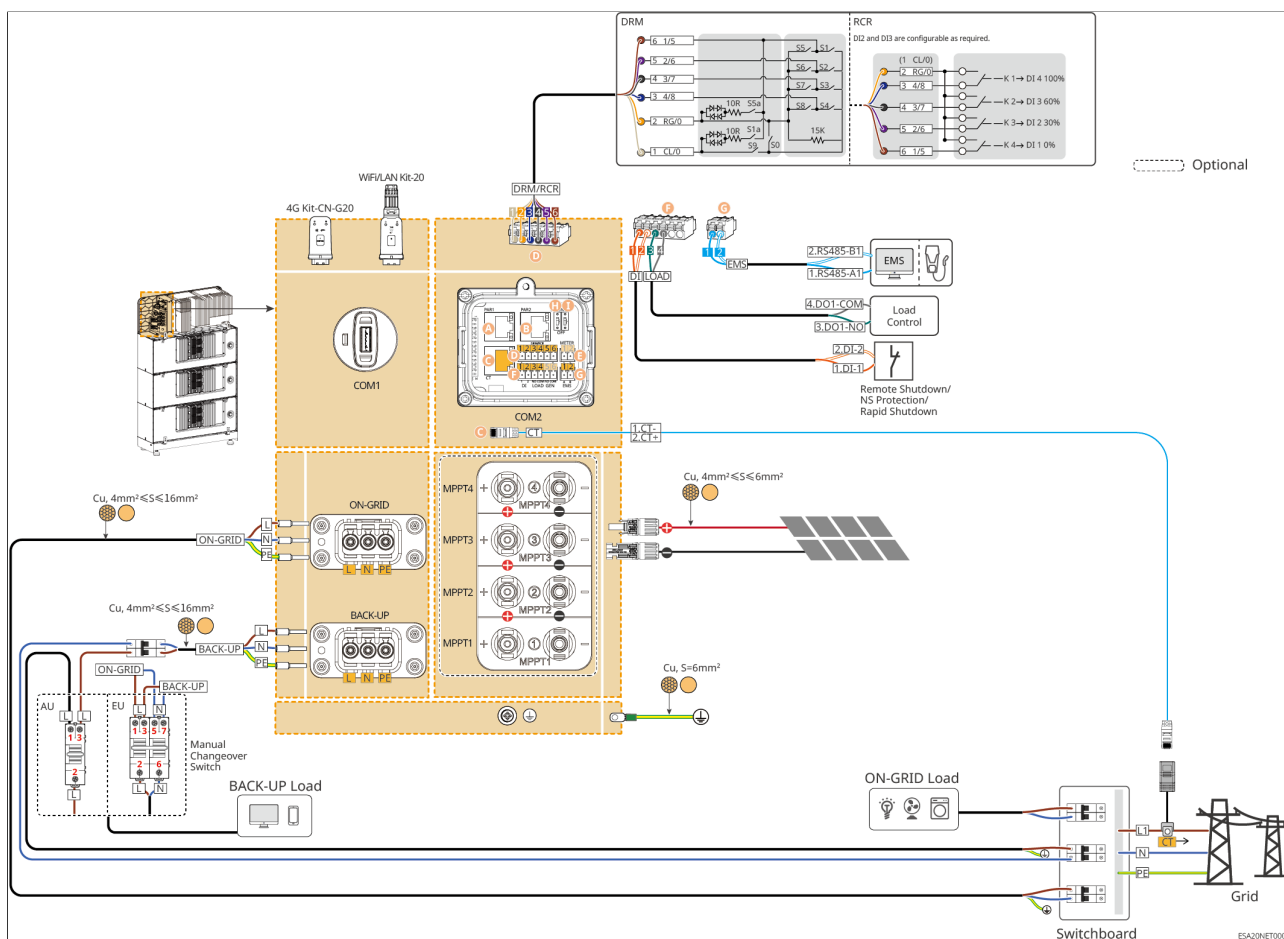
Figuur20 Scenario met ingebouwde meter
