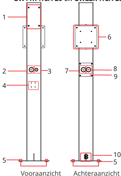
Vooraanzicht Achteraanzicht
