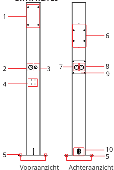
Vooraanzicht Achteraanzicht
